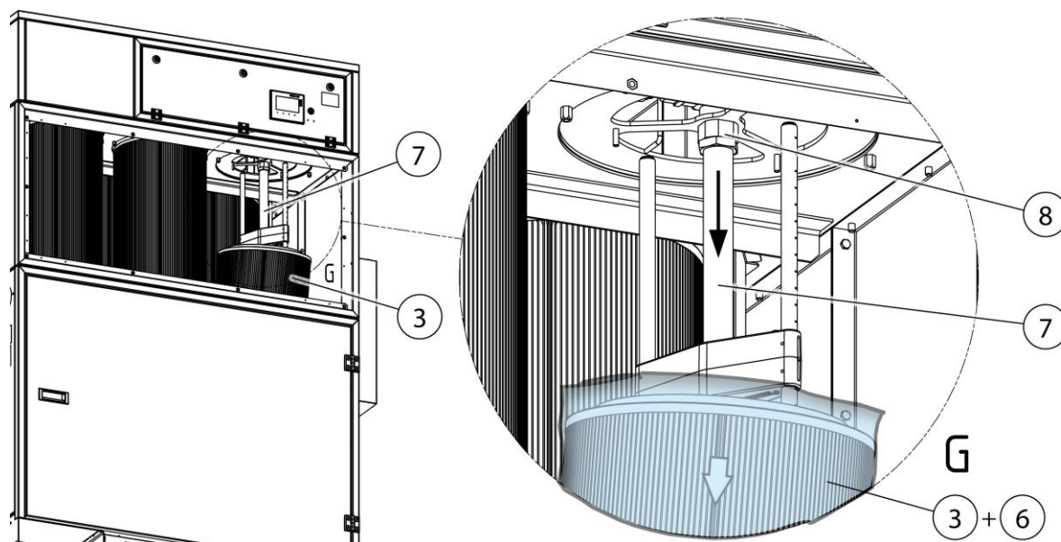
Fig. 63 : Démontage de la buse rotative
