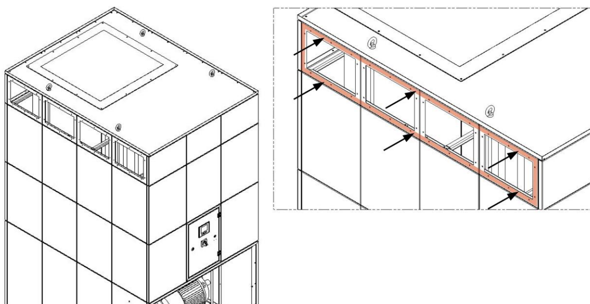
Fig. 12 : passage de l'air pur
