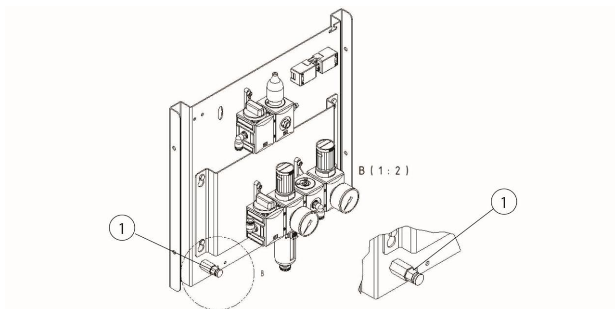
Fig. 70 : soupape de vidange des condensats réservoir d'air comprimé
