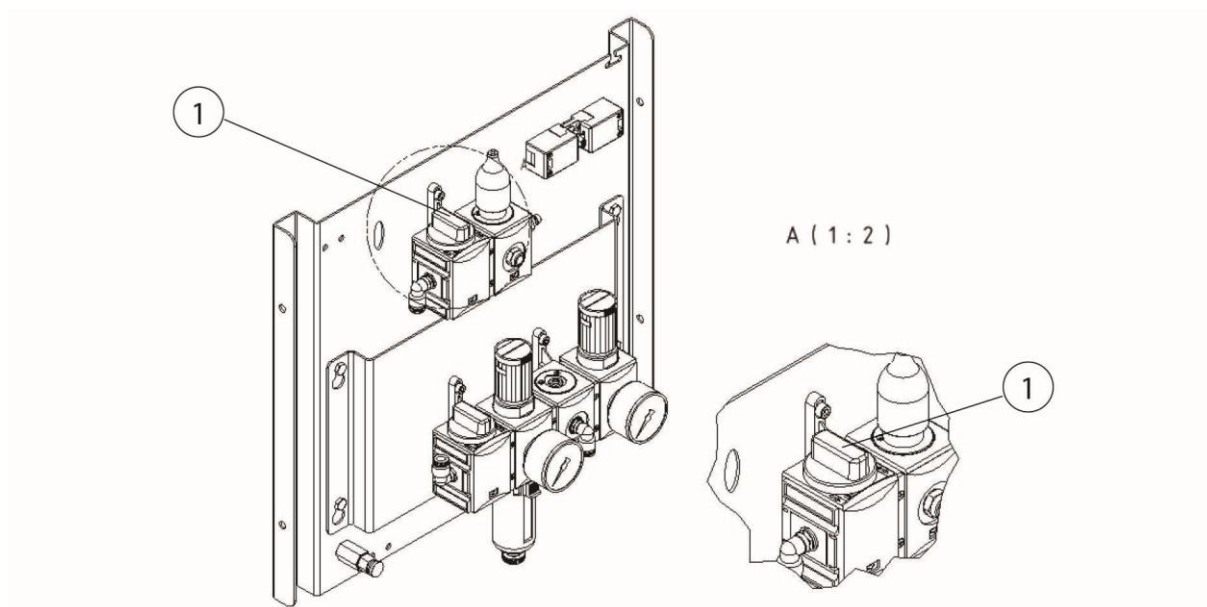
Fig. 55 : soupape pneumatique bac collecteur de poussières
