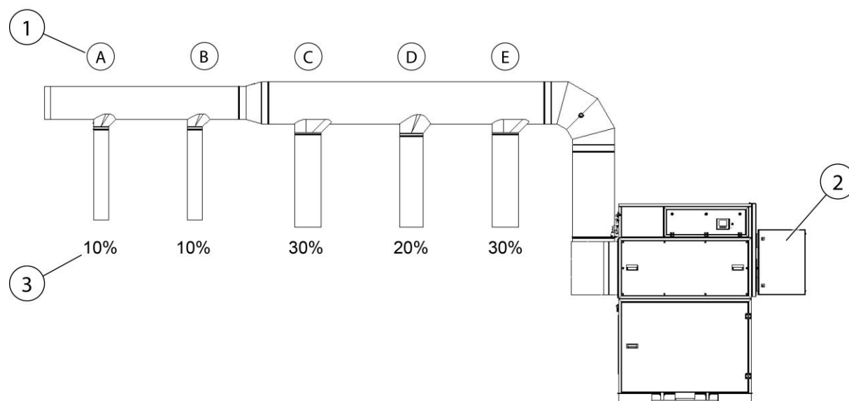
Fig. 54 : réglage de la régulation de la puissance d'aspiration
