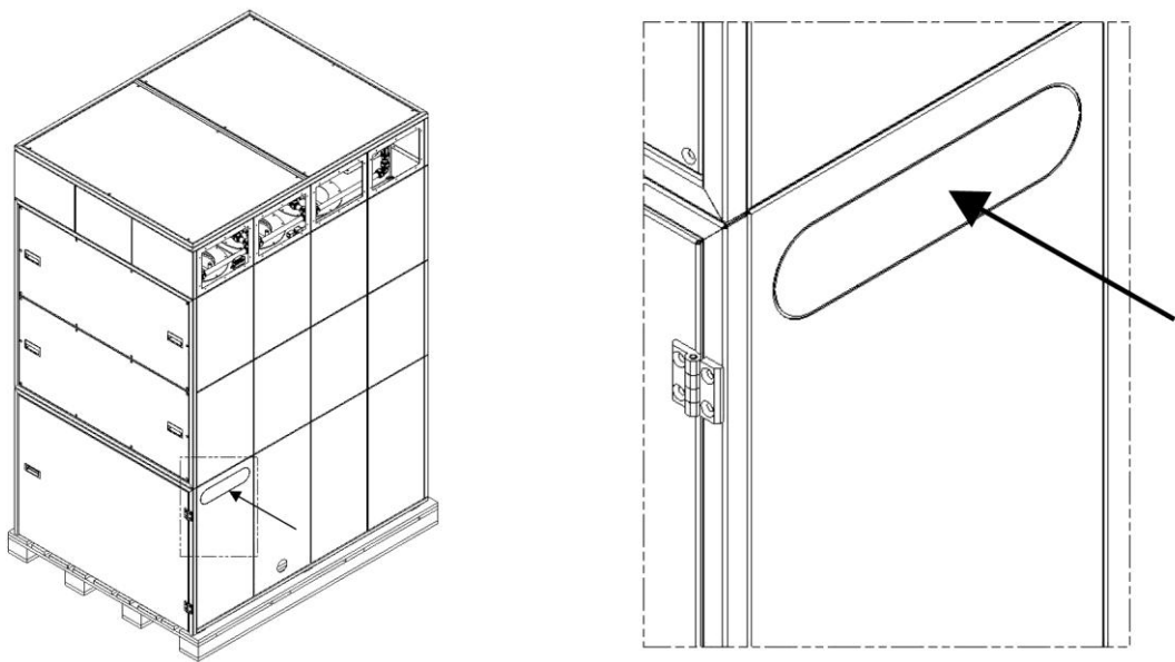
Fig. 13 : tôle à trous oblongs
