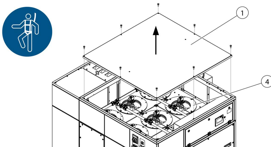
Fig. 64 : Remplacement du filtre – Démontage de la tôle de recouvrement
