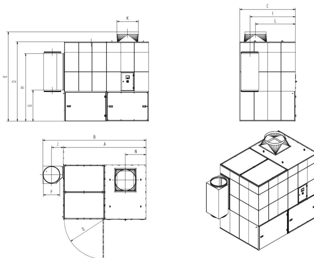
Fig. 76 : Fiche dimensionnelle 34130
