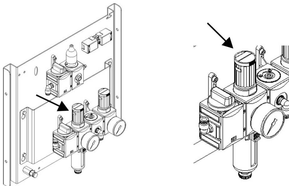
Fig. 29 : réglage de la pression de service
