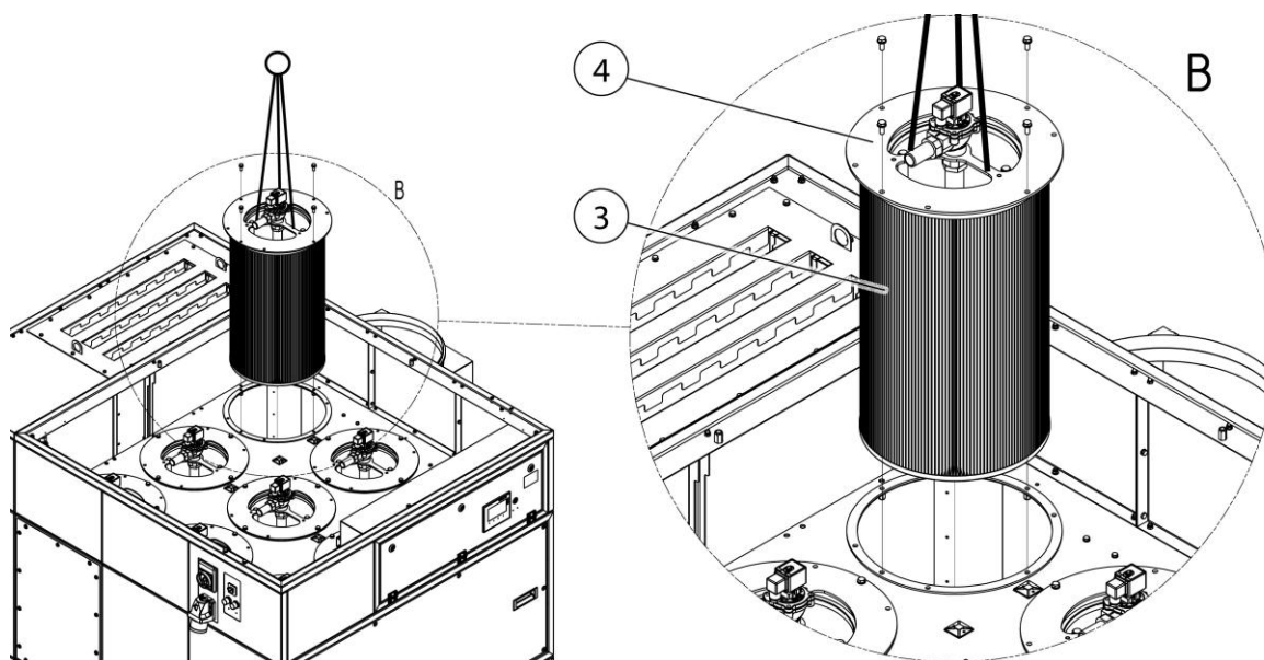
Fig. 67 : Remplacement du filtre – Démontage du porte-filtre
