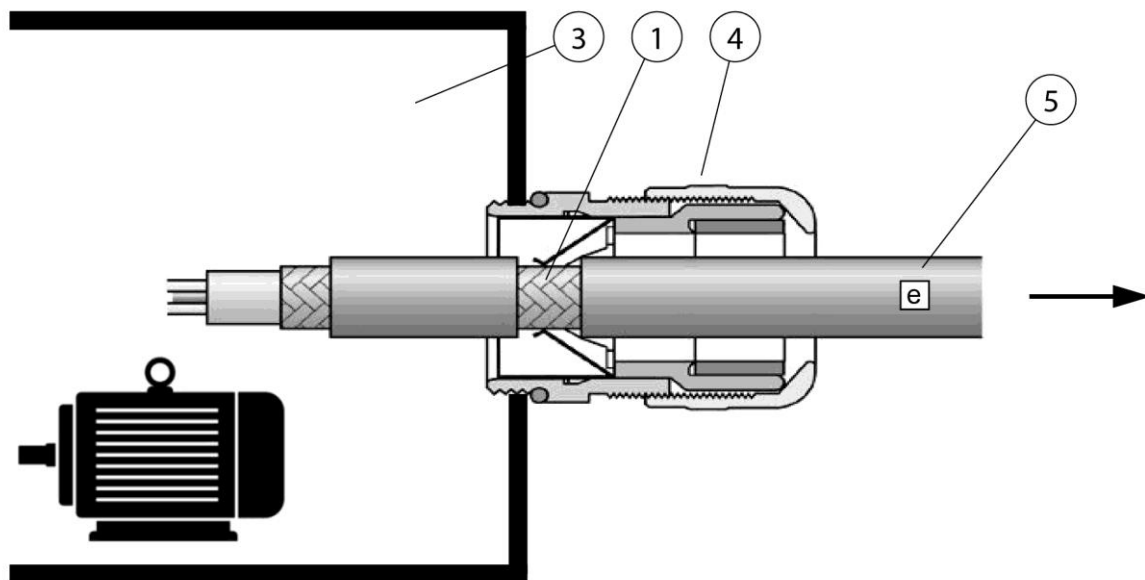
Fig. 37 : raccordement du blindage du câble du moteur
