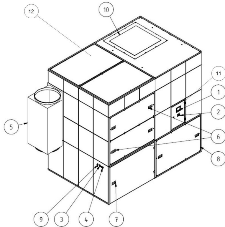
Fig. 1: 34110 - 34130
