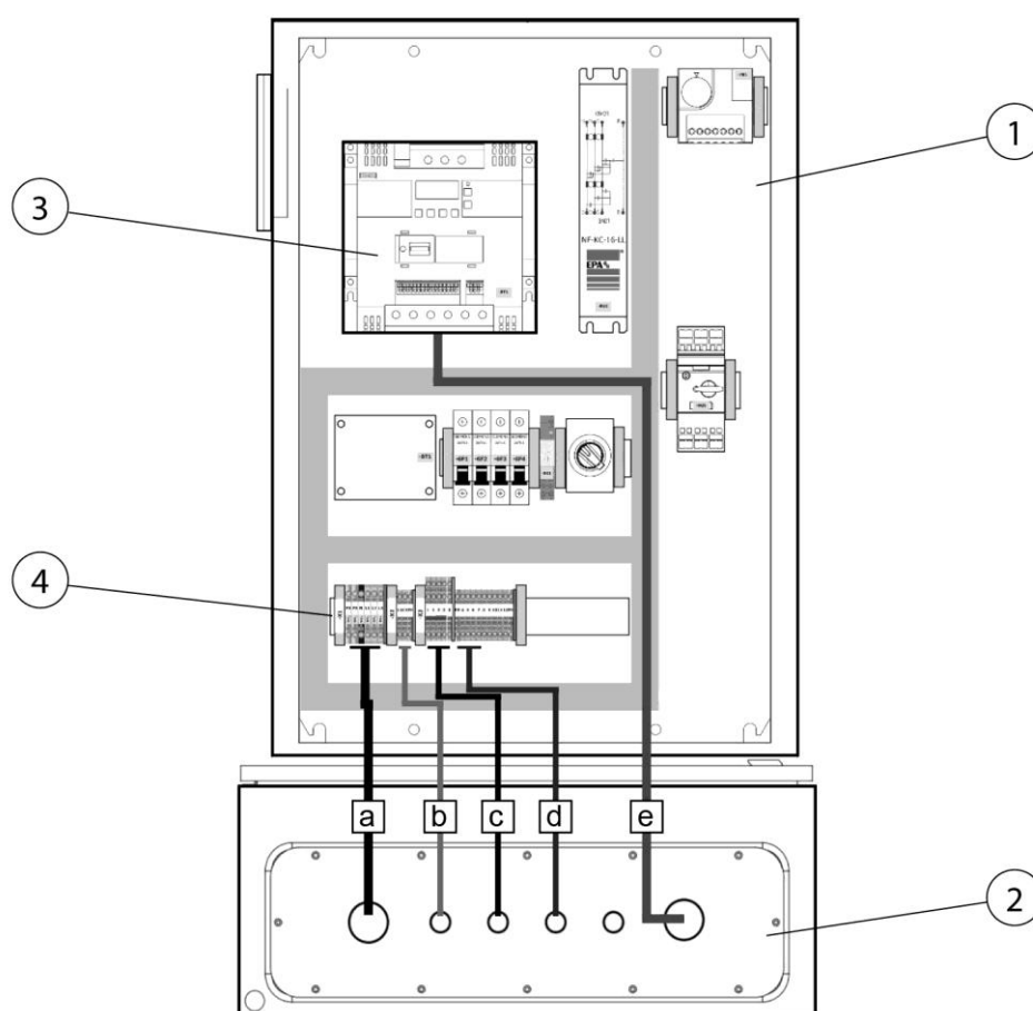
Fig. 34 : armoire de commande régulation de la puissance d'aspiration
