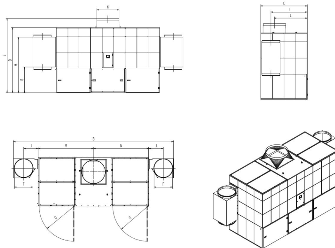
Fig. 78 : Fiche dimensionnelle 34180
