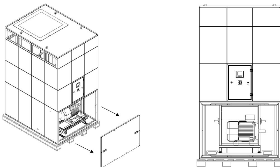
Fig. 9 : ouverture de la porte de maintenance de la section du ventilateur
