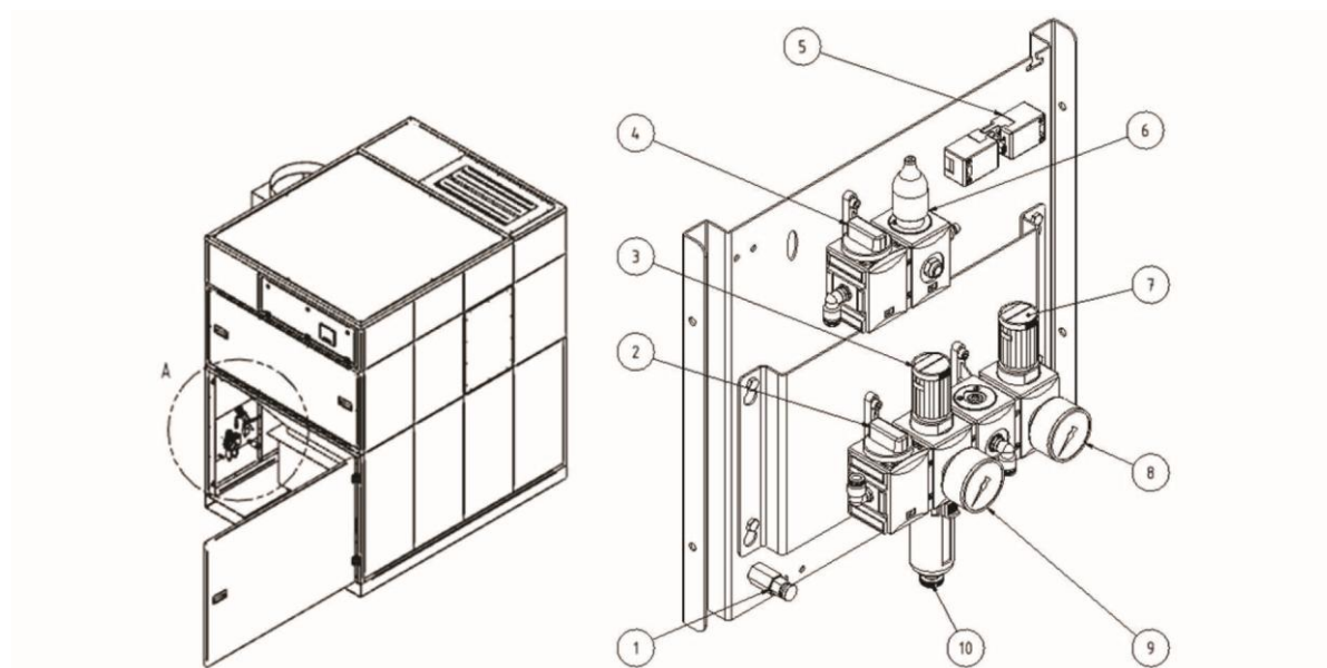
Fig. 27 : l'unité d'air comprimé
