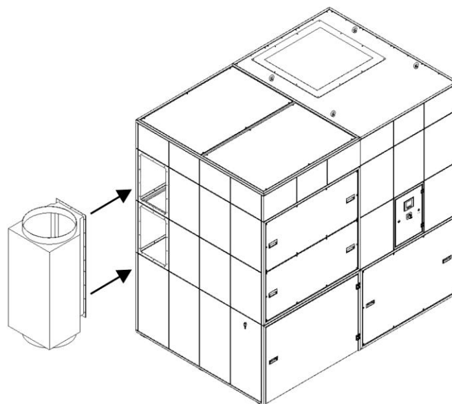
Fig. 26 : montage du boîtier de raccordement côté aspiration
