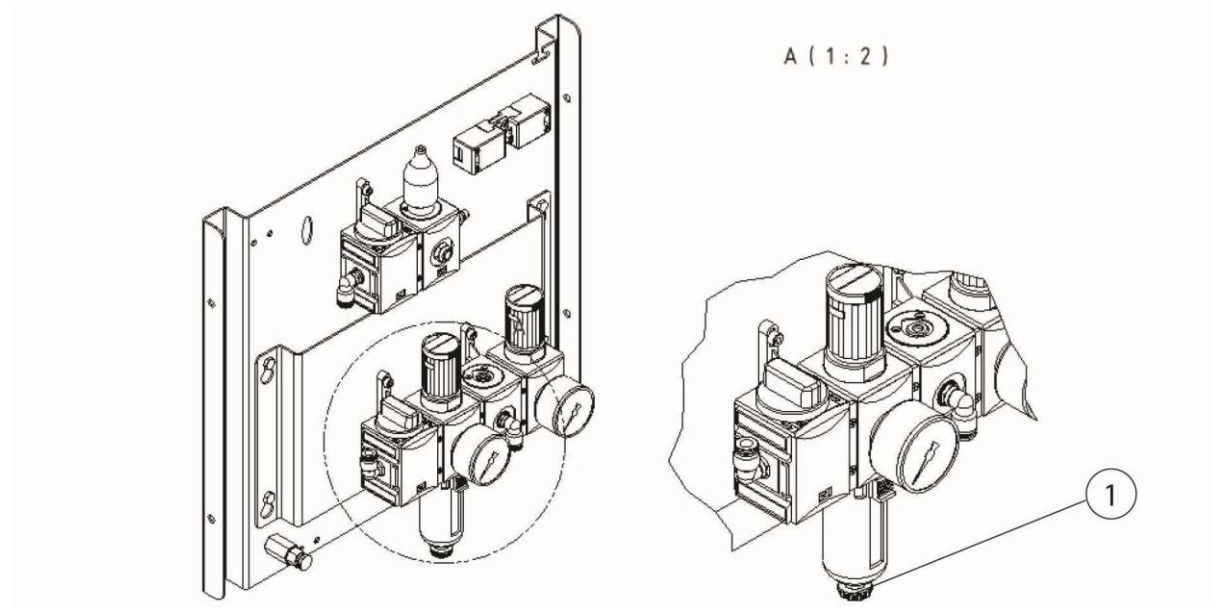
Fig. 71 : soupape de vidange des condensats unité de maintenance d'air comprimé
