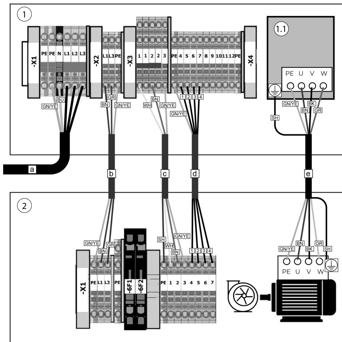
Fig. 35 : schéma de câblage de la régulation de la puissance d'aspiration avec produit
