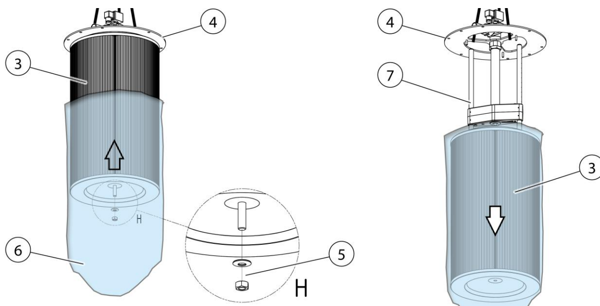
Fig. 68 : Remplacement du filtre – Démontage de la cartouche filtrante
