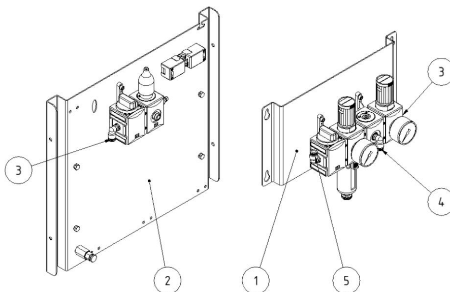
Fig. 31 : l'unité d'air comprimé
