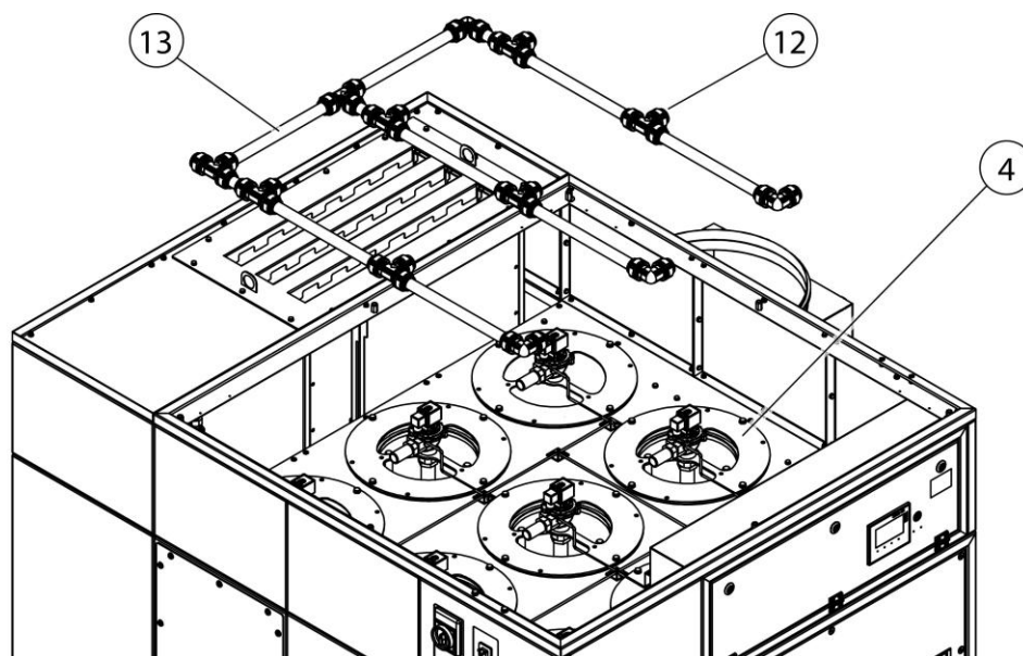
Fig. 66 : Remplacement du filtre – Démontage de la tuyauterie d'air comprimé
