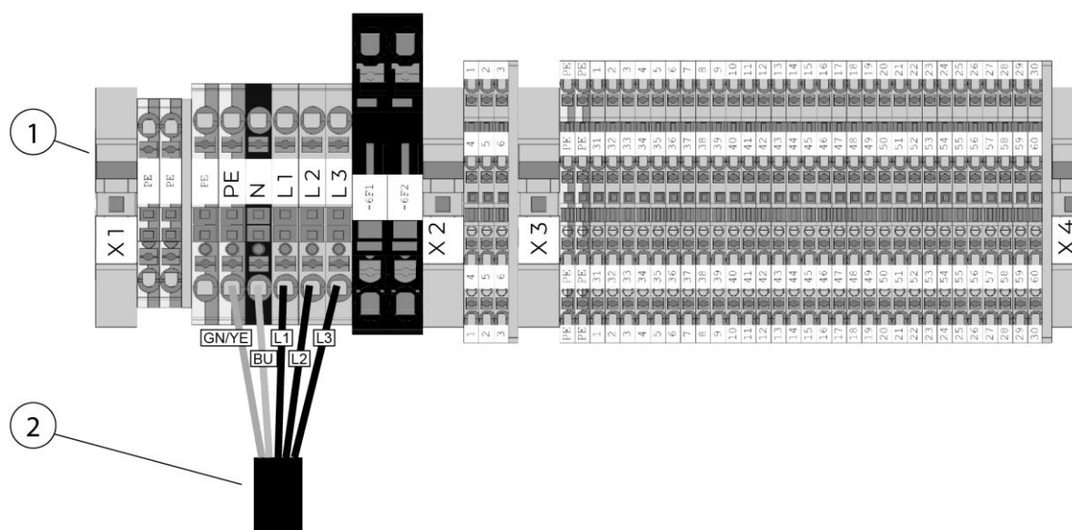
Fig. 32 : réglette à bornes de raccordement armoire de commande produit
